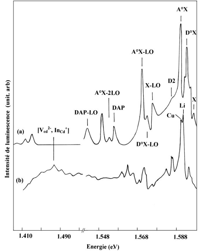
Figure 2: Spectre de photoluminescence à basse température pour la face Te. Etat indenté. (a) Etat non indenté, (b) Etat indenté.
