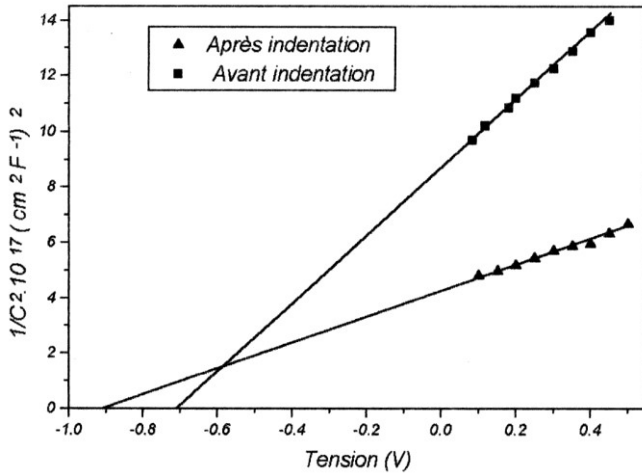
Figure 3 : Caractéristique (1/C^2) -V de la face Cd.
