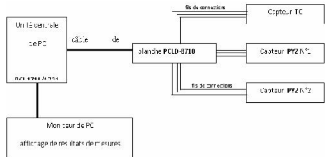
Figure 2 : Montage réalisé pour l'obtention des mesures par les des mesures par le logiciel « Advantech GeniDAQ Demo »
