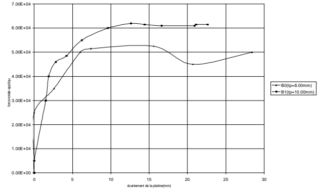
Figure 4 : Force totale appliquée en fonction de l'écartement de la platine-influence de l'épaisseur de la platine pour les assemblage raidis
