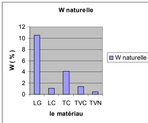
Figure 2 : Teneur en eau initiale des différents matériaux
