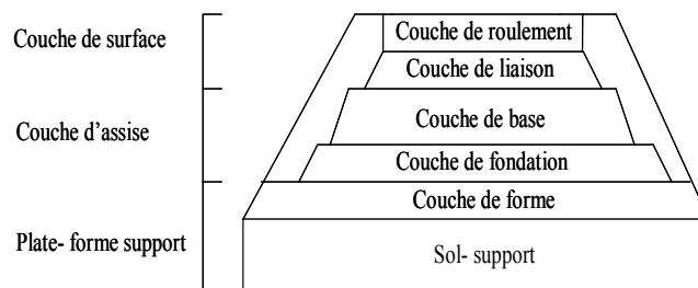
Figure 1 : Constitution d'une structure de chaussée
