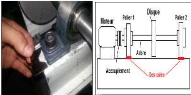
Figure.5. Position des cales pour le mauvais alignement
