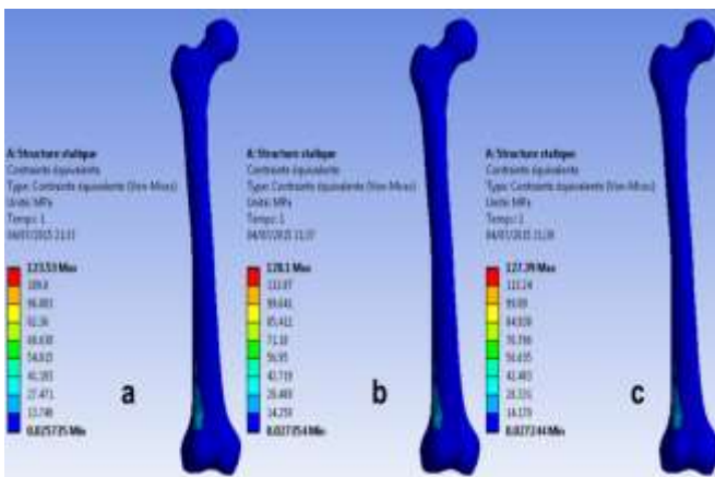
Figure 6 : Contrainte équivalente (Von Mises) de fémur humain orthotrope
