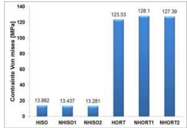
Figure 7 : Comparaison des résultats des contraintes
