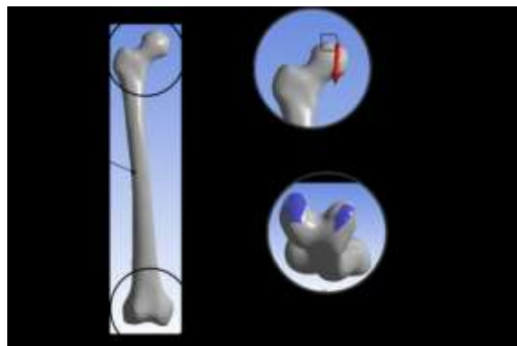
Figure 4 : Conditions limites et chargement
