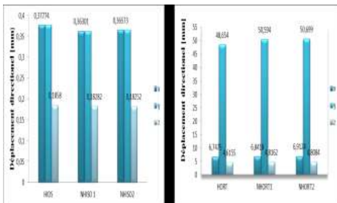
Figure 10: Comparaison des résultats des déplacements
