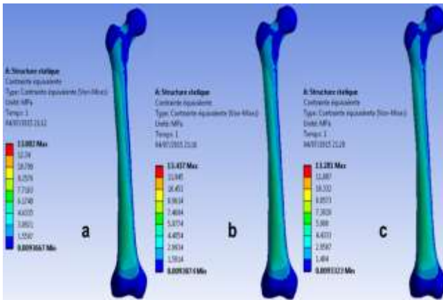
Figure 5 : Contrainte équivalente (Von Mises) de fémur humain isotrope.
