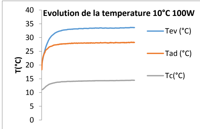
Figure 7 : Comportements de la température du caloduc en position horizontale
