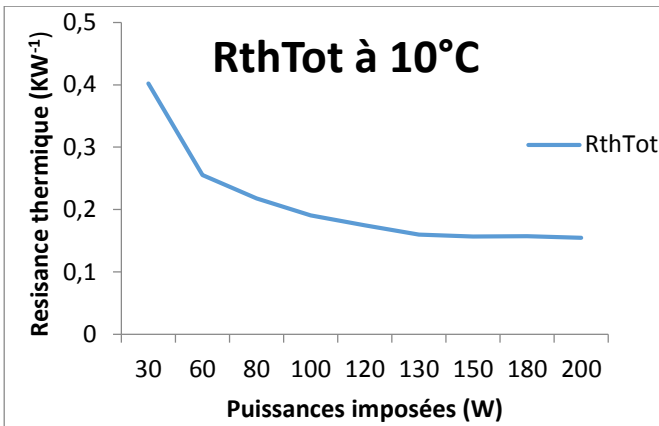
Figure 10 : Effet de la puissance sur la résistance thermique totale
