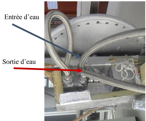
Figure 6: Circuit de refroidissement d'eau
