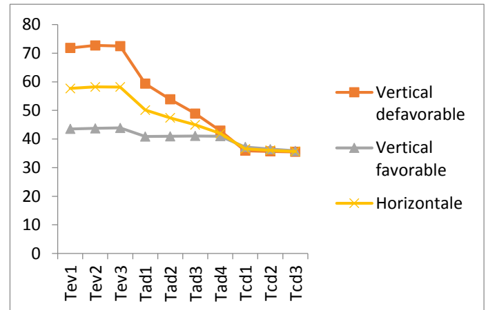
Figure 12 : Distributions axiales de température à 35°C imposées 30W
