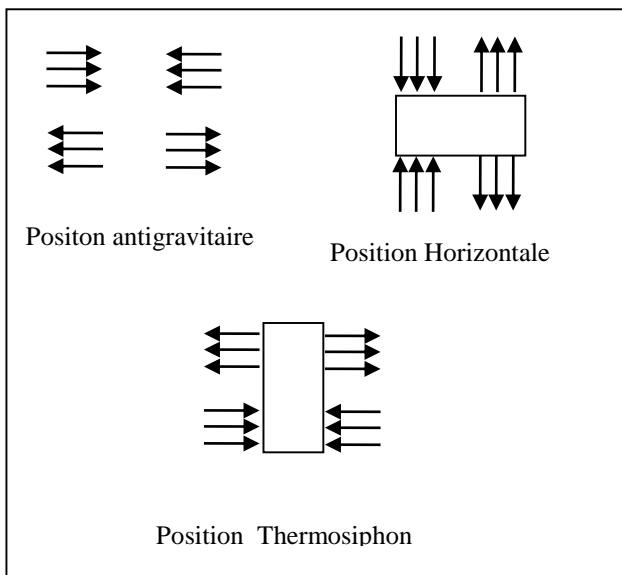
Figure 11 : Différentes positions expérimentées
