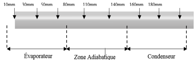
Figure 5 : Position des thermocouples le long du caloduc
