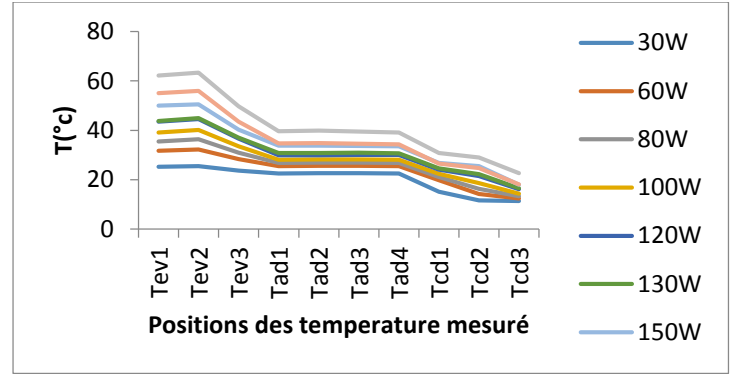
Figure 8 : Distribution axiale de la température en fonction de différentes puissances imposées
