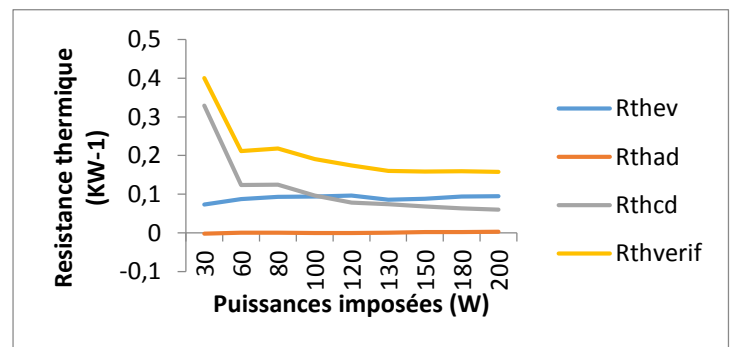
Figure 9 : Effet de la puissance sur les résistances thermiques
