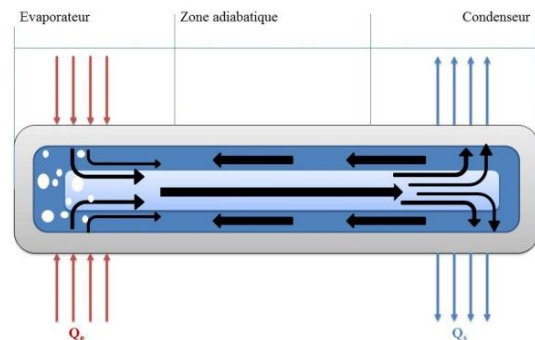
Figure 1 : Principe de fonctionnement d'un caloduc
