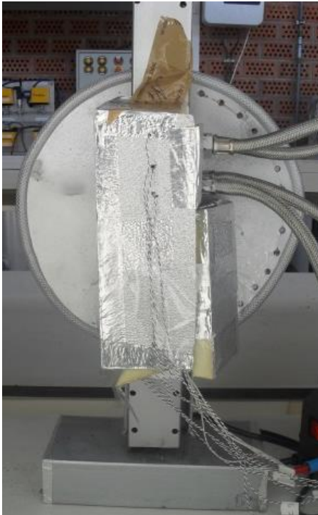
Figure 3 : Le caloduc installé sur le support tournant pour changement de positions
