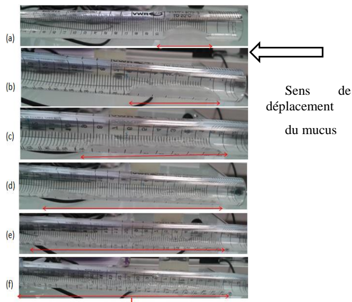
Figure 2: Transport du mucus synthétique à une fréquence de 9Hz en fonction des dépressions (a) 0%, L= 3,2 cm, (b) 10%, L=5,2 cm, (c) 15%, L=8 cm, (d) 25%, L=11,2 cm, (e) 40%, L=14,3 cm et (f) 50%, L=17,3 cm.
