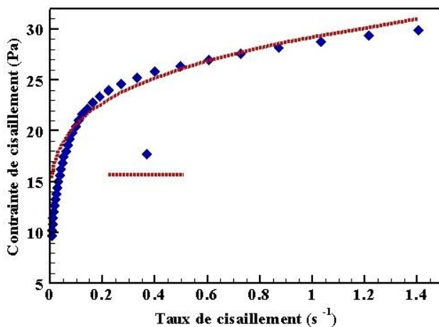
Figure 7: comparaison du rhéogramme d'un mucus synthétique à 1,5 g d'Actigum, Avec celui obtenu avec le modèle d'Herschel-Bulkley à T= 20°C
