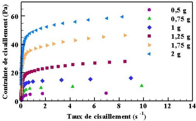
Figure 4: Variation de la contrainte de cisaillement en fonction du taux de cisaillement pour différentes concentrations à T=20°C
