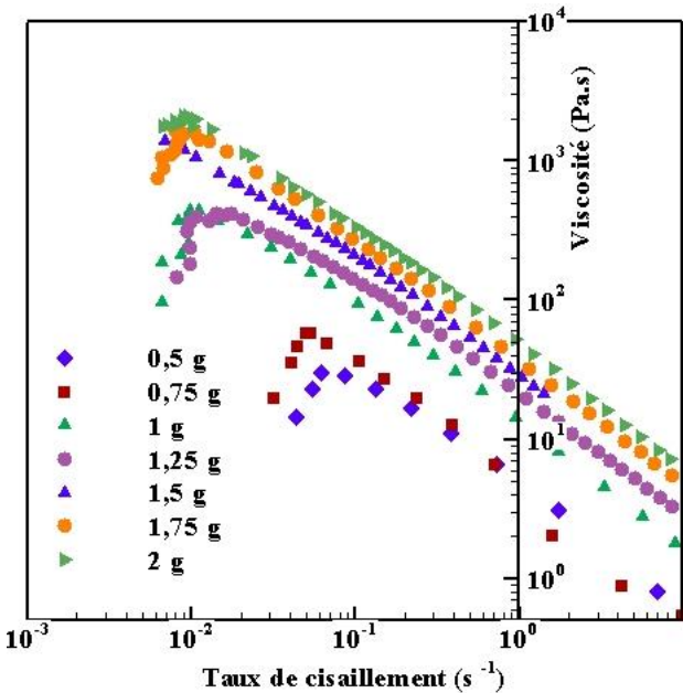
Figure 5: Courbe de viscosité pour différentes concentrations à T=20°C
