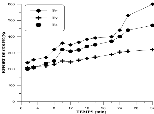
Figure 4 : Evolution des efforts de coupe en fonction du temps d'usinage V c = 180 m/min ; a p = 0,5 mm ; f = 0,08 mm/tr.
