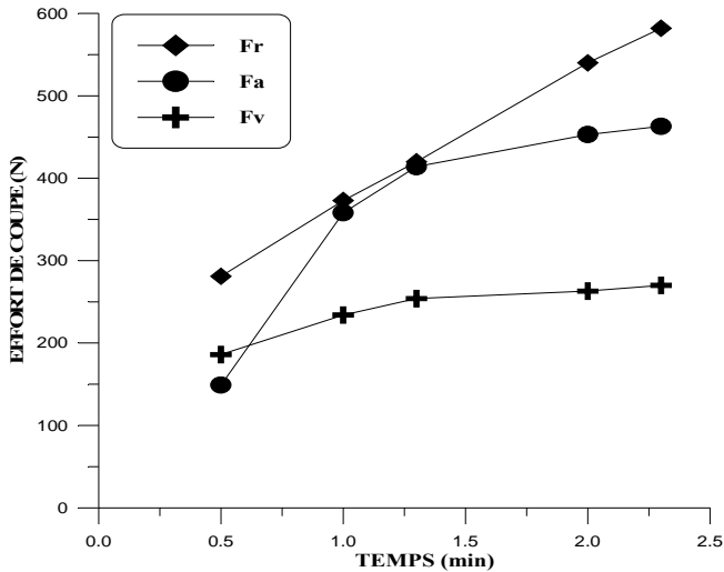
Figure 6 : Evolution de l'effort de coupe en fonction du temps d'usinage V_c = 350 m/min; a_p = 0,5 mm; f = 0,08 mm/t
