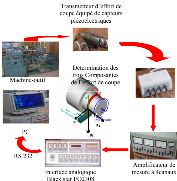
Figure 1 : Dynamomètre pour la mesure des efforts de coupe
