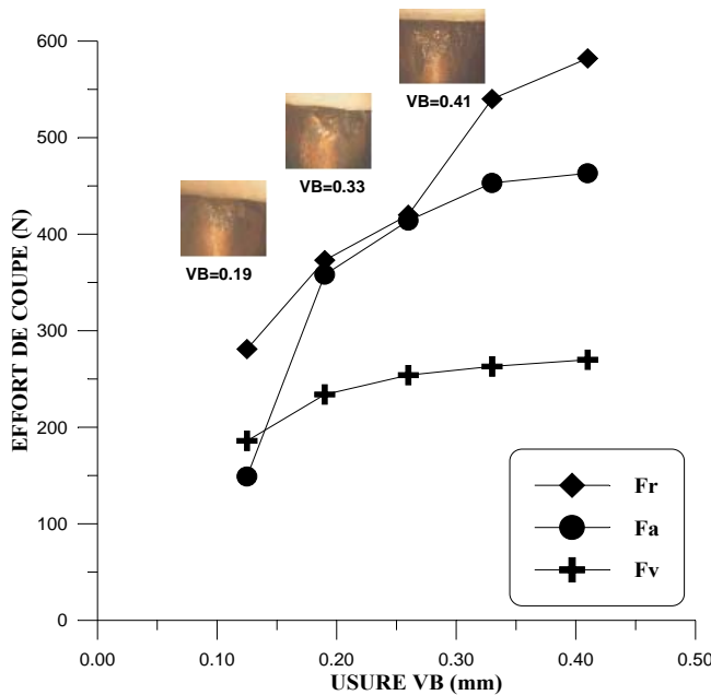
Figure 7 : Evolution de l'effort de coupe en fonction de l'usure V_c = 350 m/min; a_p = 0,5 mm ; f = 0,08 mm/tr
