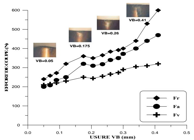
Figure 5 : Evolution des efforts de coupe en fonction de l'usure V c = 180 m/min ; a p = 0,5 mm ; f = 0,08 mm/tr
