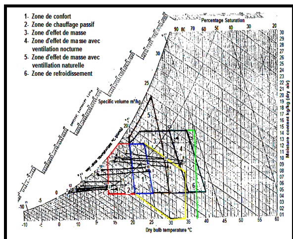
Fig. 3 : Diagramme psychrométrique de S.ZOCHOLAY appliqué à la ville de Constantine. Source : Auteur
