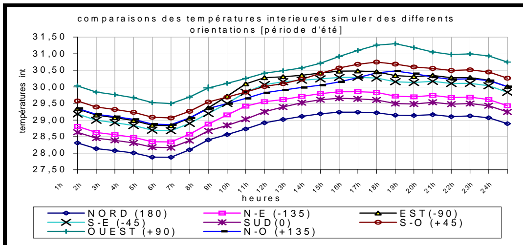
fig.13 : Effet de l'orientation sur la température intérieure [période d'été]
