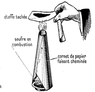
Décoloration par le gaz sulfureux
